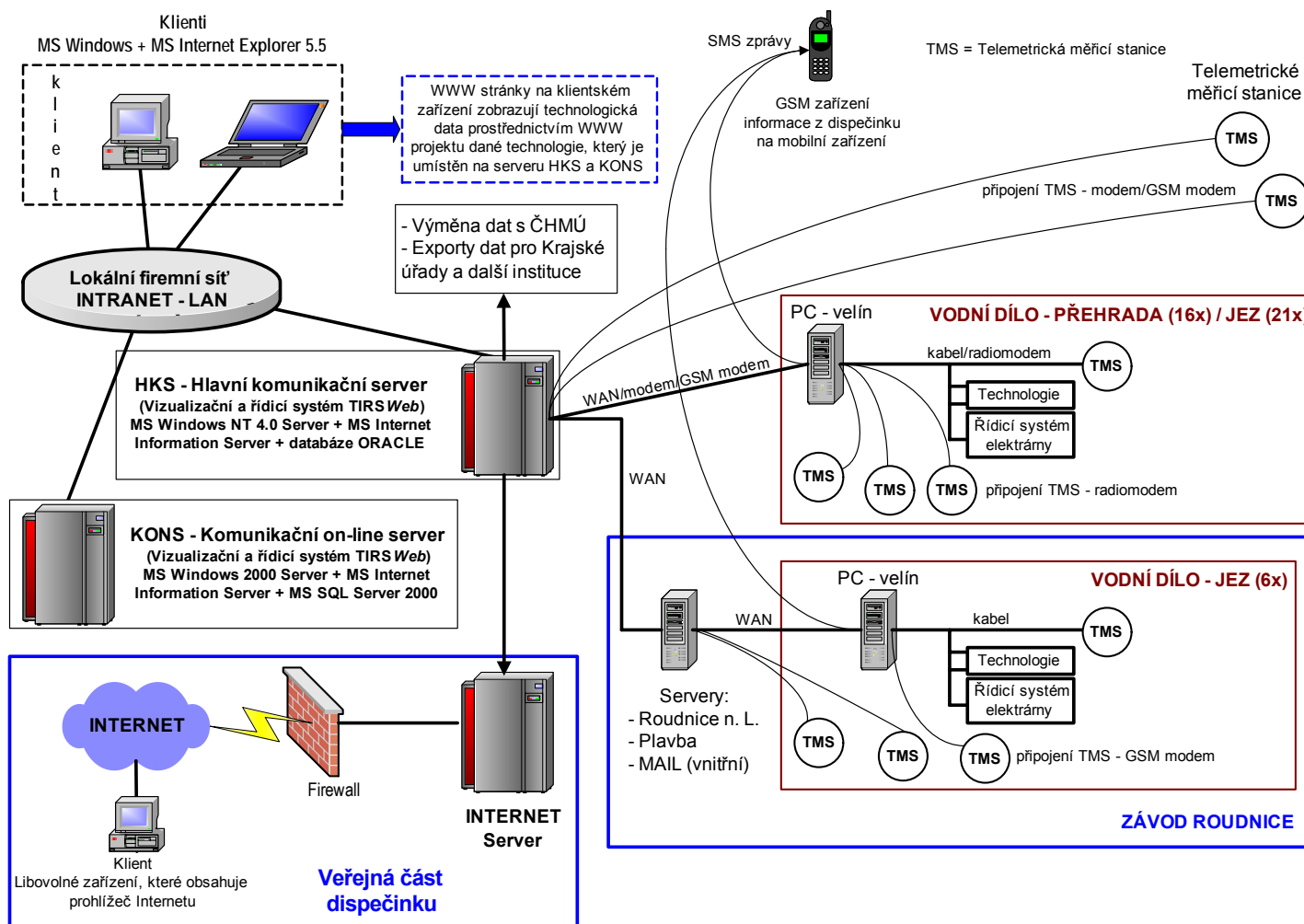
Obr. 2 - Povodí Labe, s.p. - zjednodušená topologie VHD dispečinku
